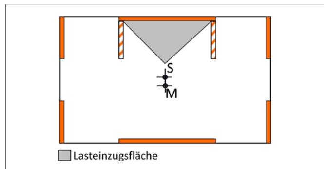
Abbildung 4.2: Grundriss mit kurzen vertikal tragenden Wänden im Bereich schubbeanspruchter Wände
