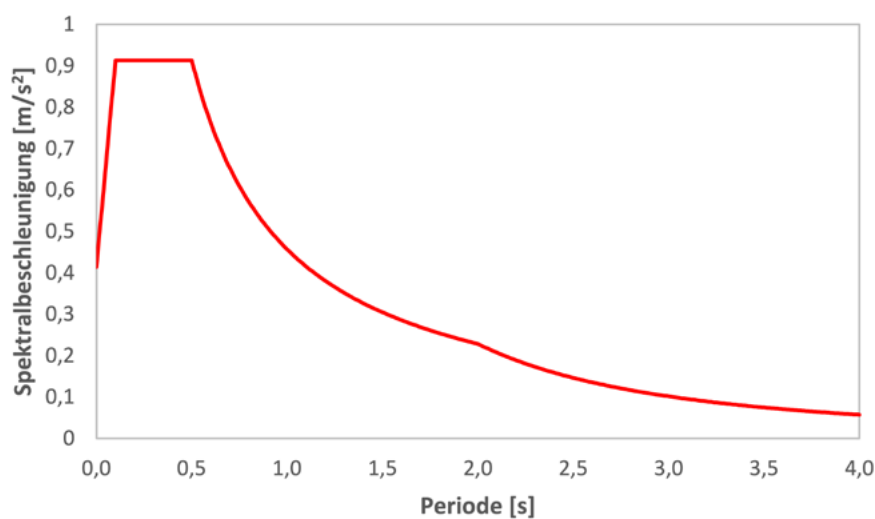
Abbildung 7.11: Bemessungsspektrum ( S_{aPR} = 1,35 \text{ m/s}^2 , Untergrundkombination C-S, q = 1,7 )
