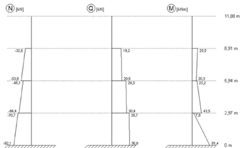
Abbildung 7.12: Schnittgrößenverlauf der Wandscheibe 7 für Einwirkungskombination „STAT + 1,0 SRSS-x + 0,3 SRSS-y“
