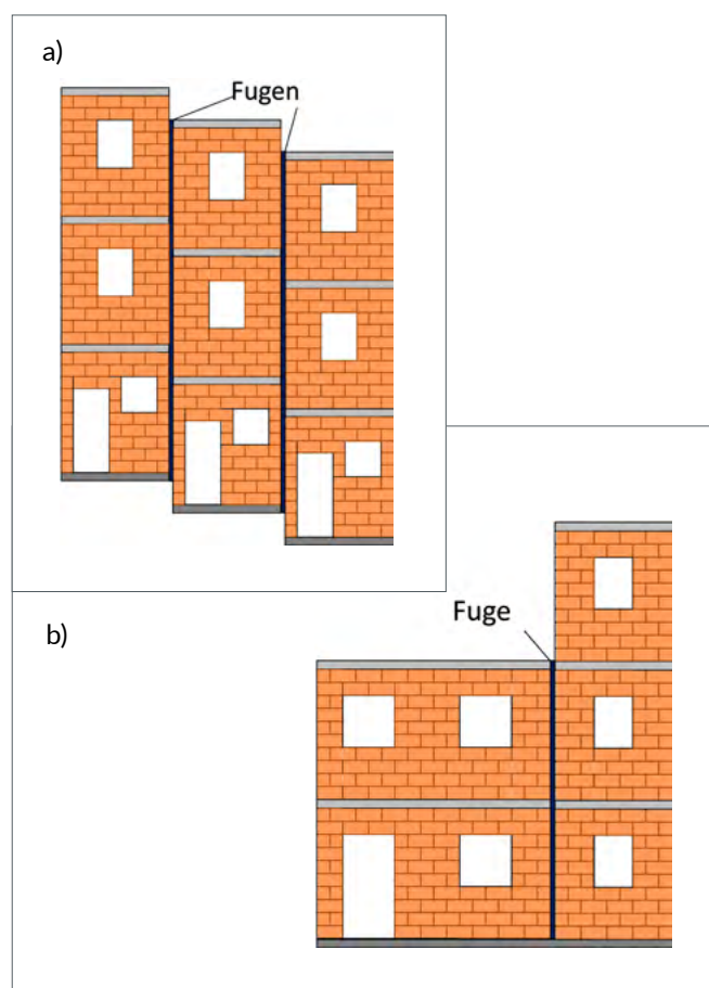
Abbildung 4.4: Fugenanordnung zwischen Gebäudeteilen mit unterschiedlichen (a) Deckenhöhen und (b) Geschosshöhen
