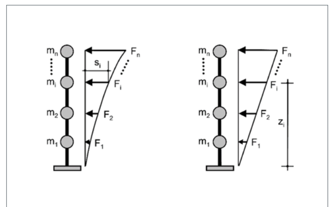
Abbildung 6.1: Verteilung der Erdbekräfte: Affin zur 1. Eigenform (links) und höhenproportional (rechts)
