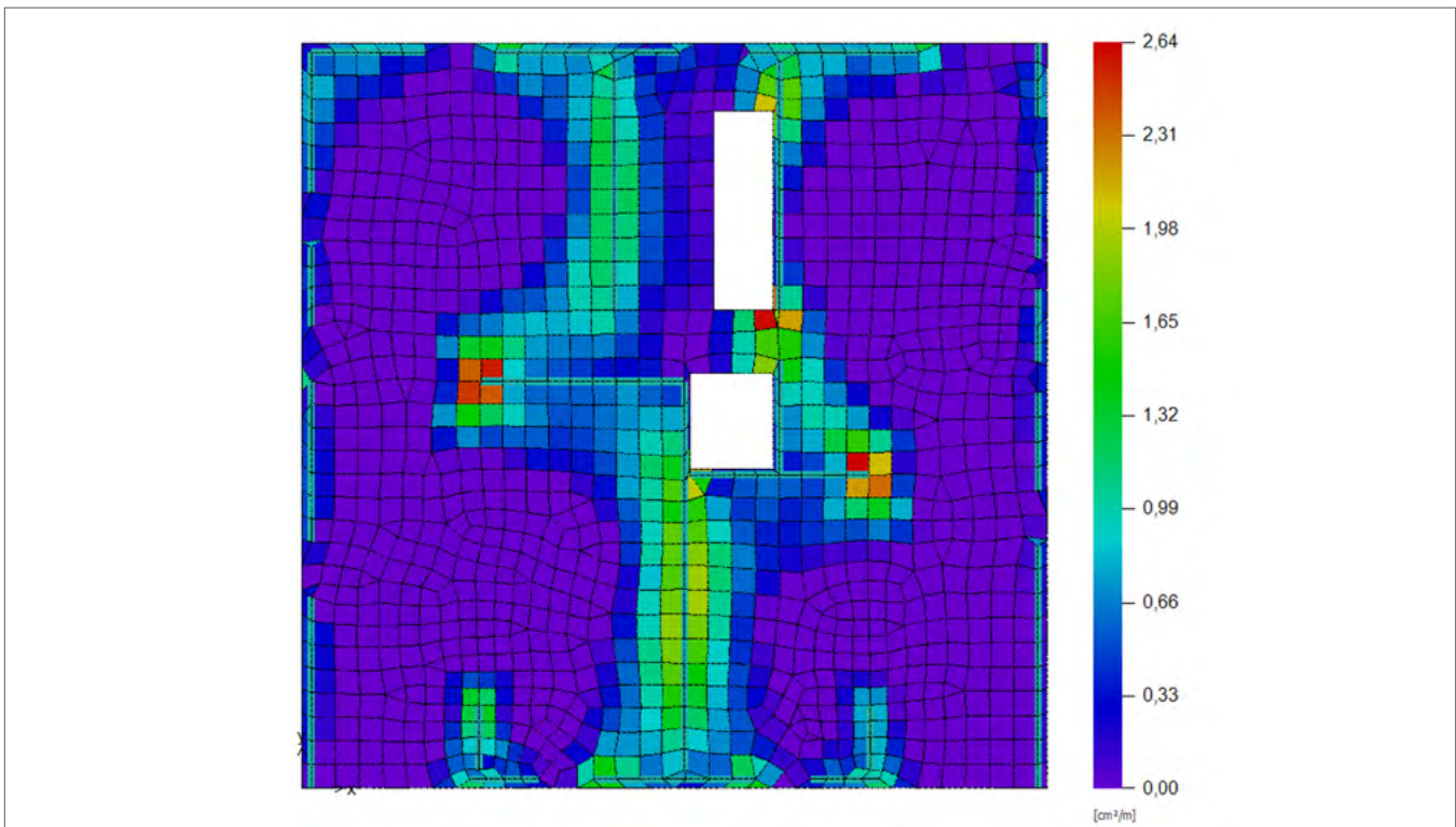
Abbildung 7.14 Erforderliche Bewehrung [cm^2/m] in der oberen Bewehrungslage der Erdgeschossdecke in x-Richtung für die Bemessungssituation Erdbeben
