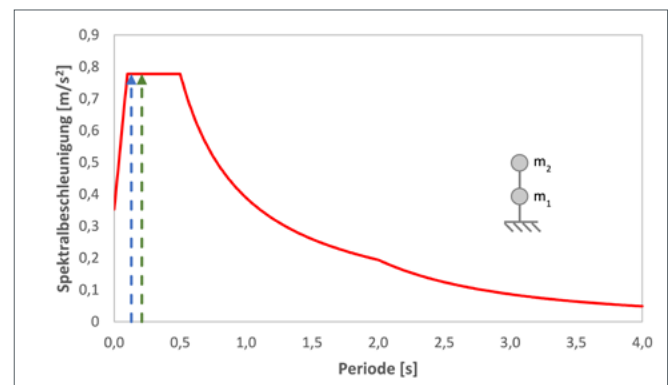
Abbildung 7.3: Bemessungsspektrum ( S_{aPR} = 1,15 \text{ m/s}^2 , Untergrundkombination C-S, q = 1,7 )
