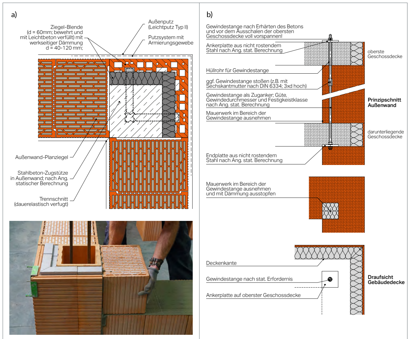
Abbildung 4.7: Rückverankerung von Decken mit geringen Auflasten: (a) Zugpfosten (b) Schlitzung mit Stabstahleinlage
