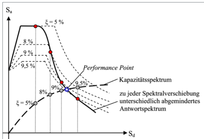
Abbildung 6.2: Ermittlung der Zielverschiebung mittels gedämpfter Spektren [15], [16]
