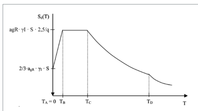
Abbildung 3.2: Horizontales Bemessungsspektrum nach DIN EN 1998-1/NA [8]
