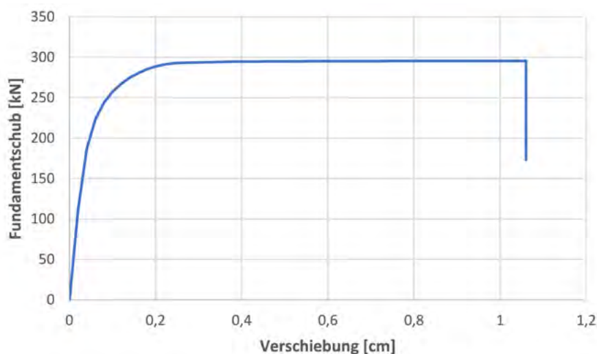
Abbildung 7.5: Gebäudekapazität für das beispielhafte Einfamilienhaus aus MINEA [18]
