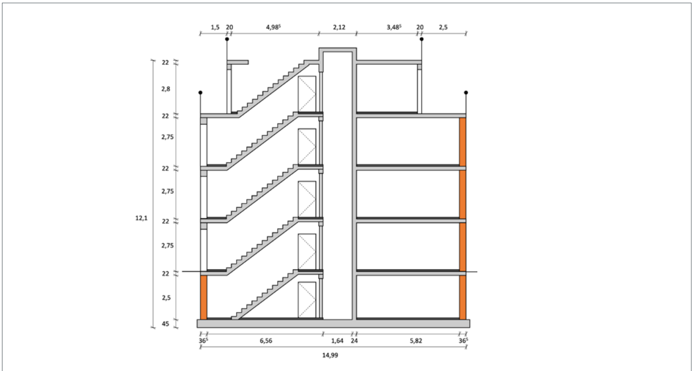
Abbildung 7.8: Schnitt A-A durch das Mehrfamilienhaus
